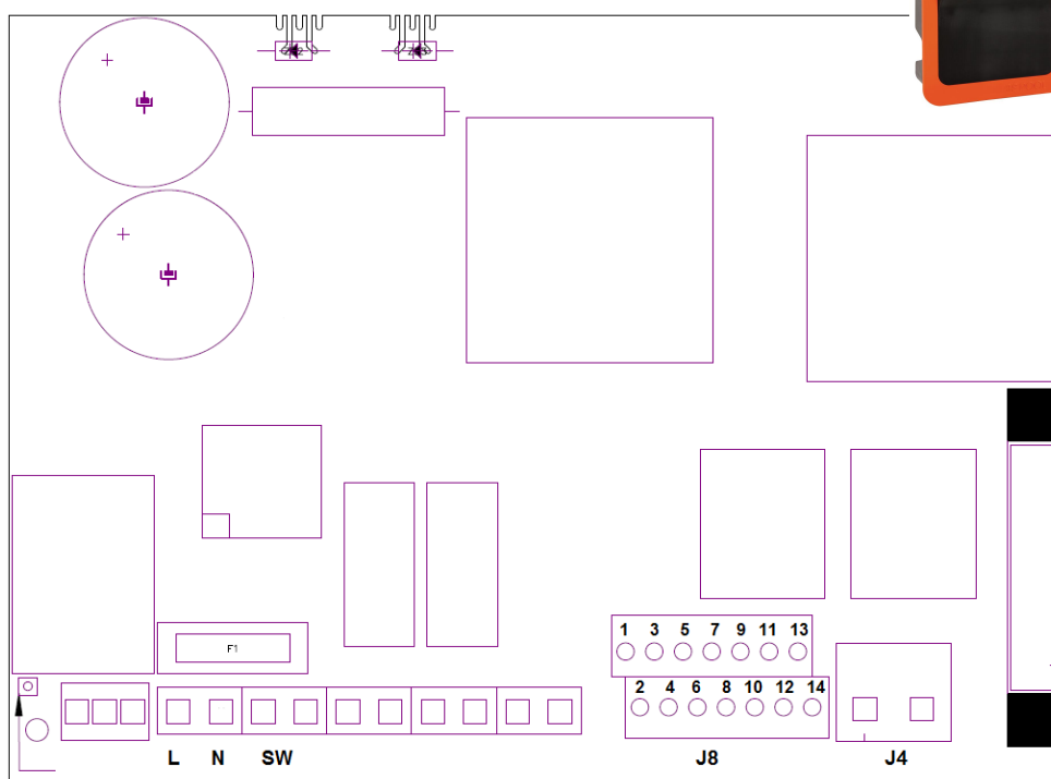
Napájecí deska -- P950/3 (10 g/h - 25 g/h) -- P953/2 (35 g/h) Měřicí deska - P909/7
